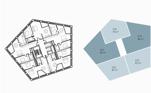
Turm 2 - 11 OG _ 1:200
