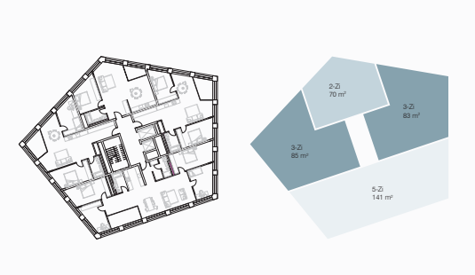
Turm 12 - 15 OG _ 1:200
