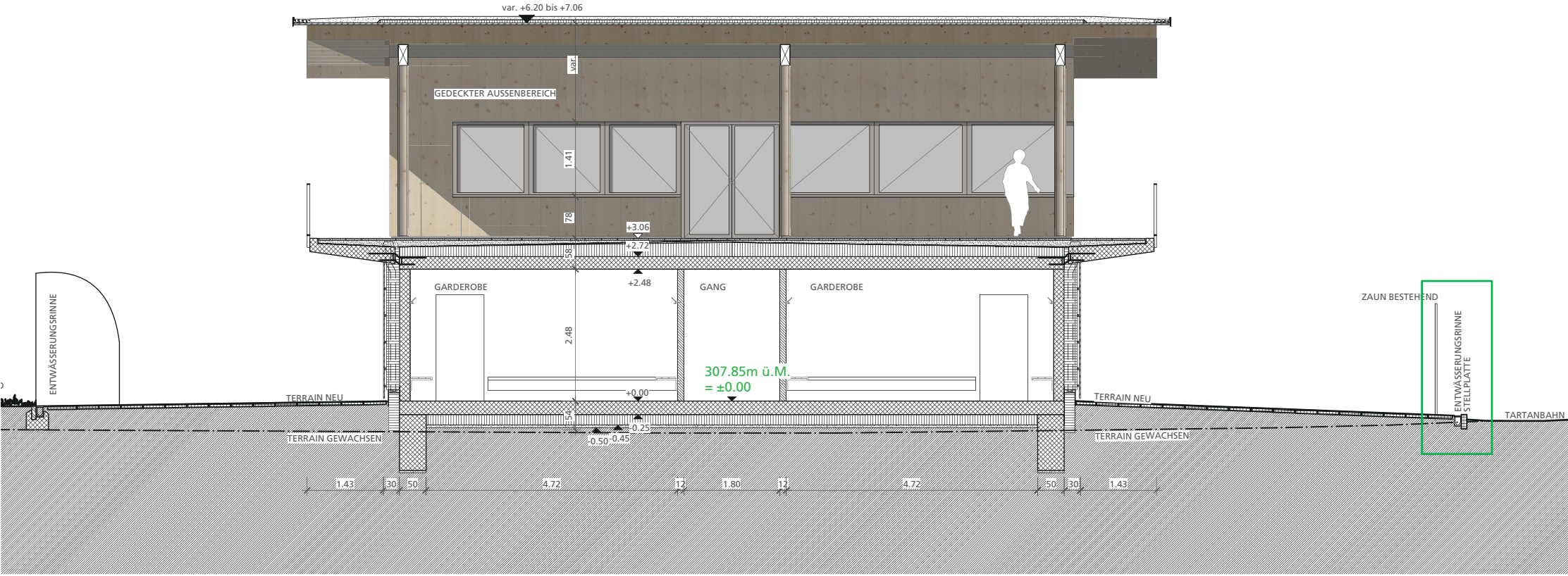
SNITT A-A
