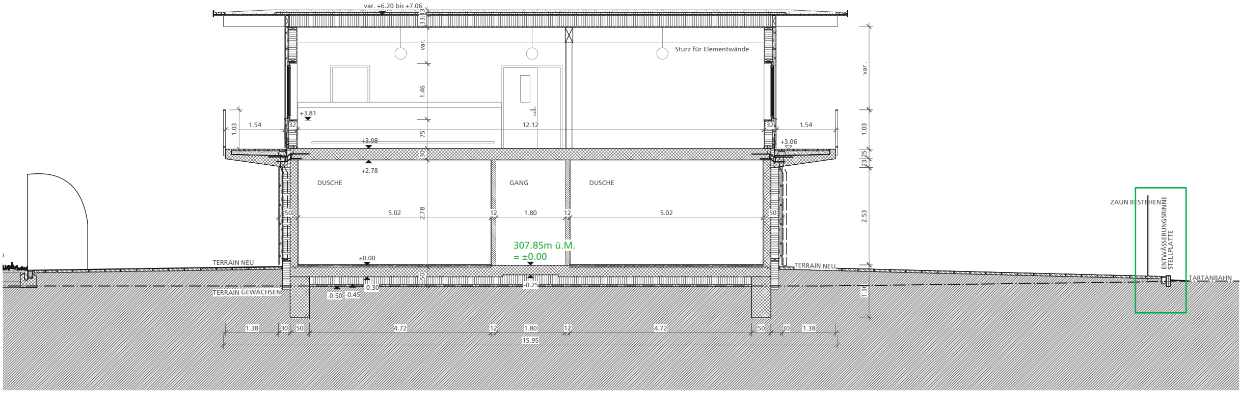
SNITT C-C
